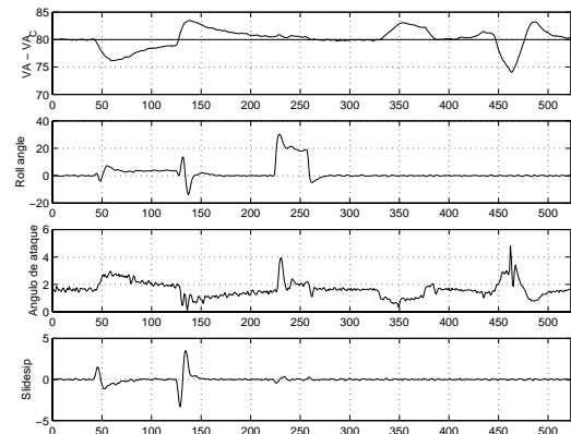
Figura 15: Velocidad, ángulos de balanceo, de ataque y de deslizamiento
