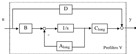
Figura 6: Estructura del prefiltro V
