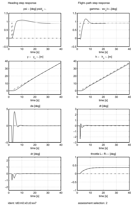
Figura 10: Respuesta a saltos en los ángulos de orientación y de rumbo
