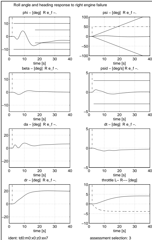
Figura 13: Comportamiento ante un fallo de motor
