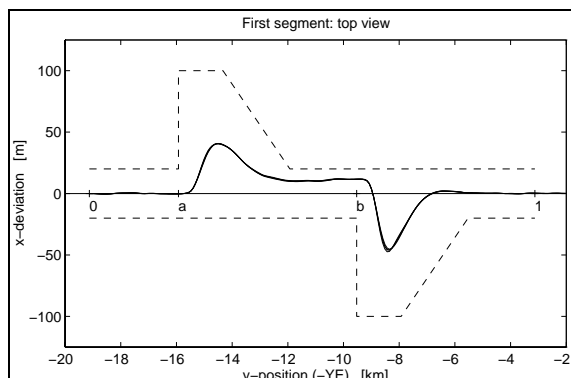
Figura 17 Efecto del fallo de motor
