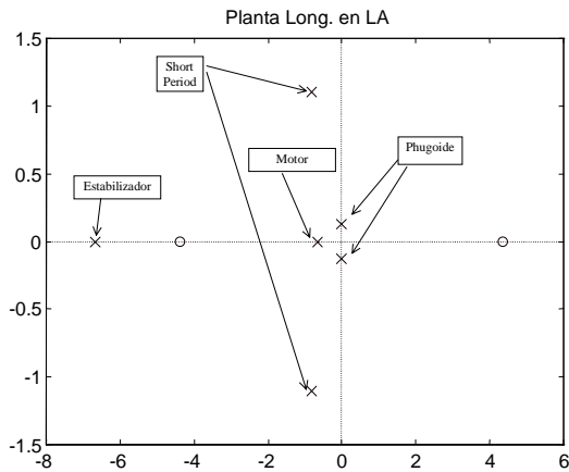
Figura 1. Polos y ceros del modelo longitudinal
