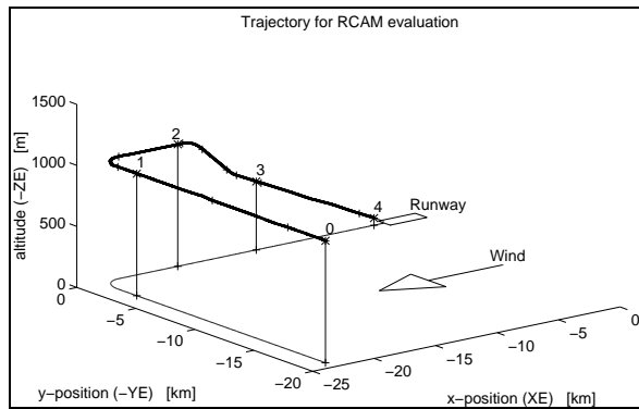
Figura 16: Trayectoria de evaluación
