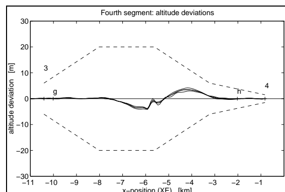
Figura 20: Aproximación final con viento racheado
