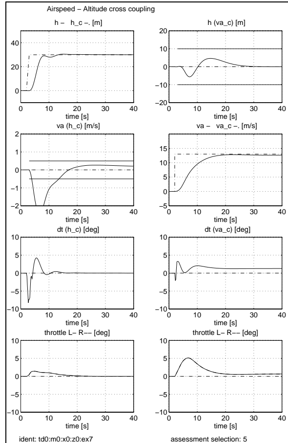
Figura 12: Salto en altura y en velocidad
