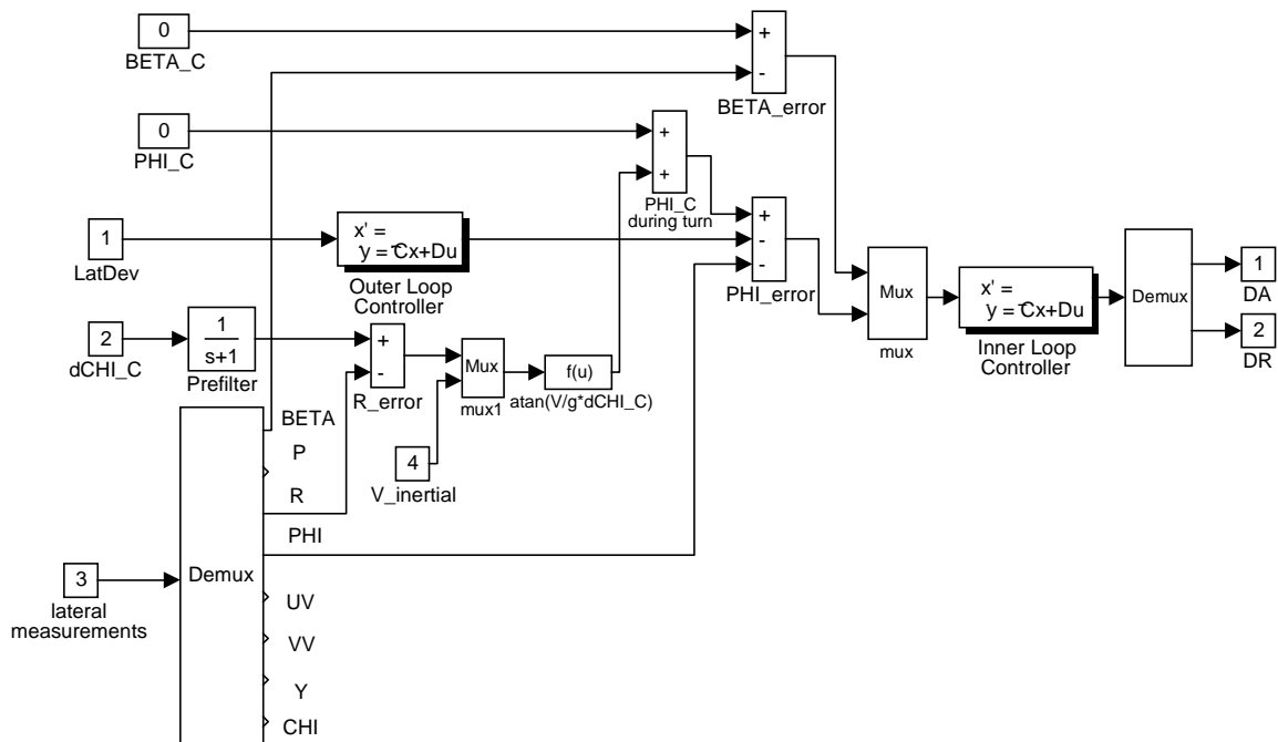
Figura 8: Estructura del controlador lateral
