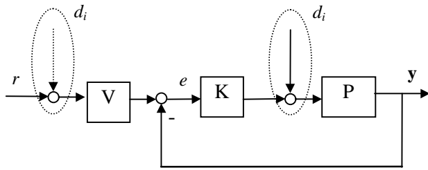
Figura 5 Diagrama de bloques con el prefiltro para la optimización de Kwakeernaak.
