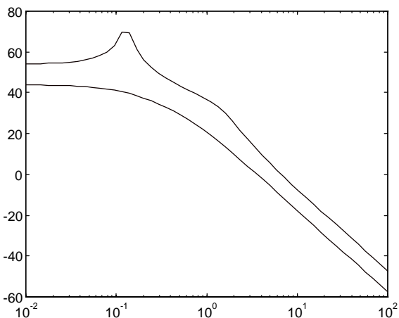
Figura 2. Valores singulares de la planta en lazo abierto = SoP
