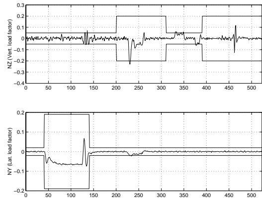
Figura 14: Aceleraciones vertical y lateral sufrida durante la trayectoria de evaluación
