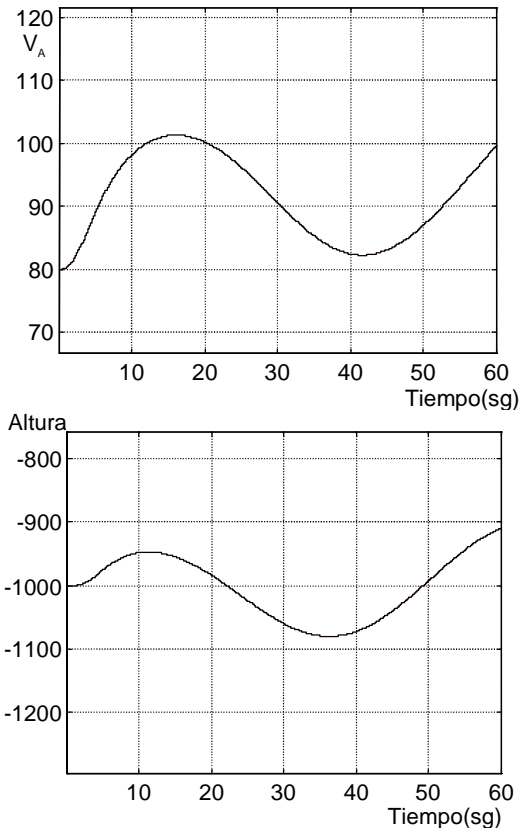
Figura 3: Respuesta a salto en VA. Simulación no lineal)
