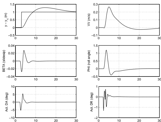
Figura 9: Desviación lateral
