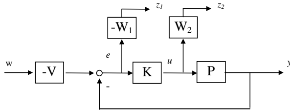
Figura 4: Planta generalizada
