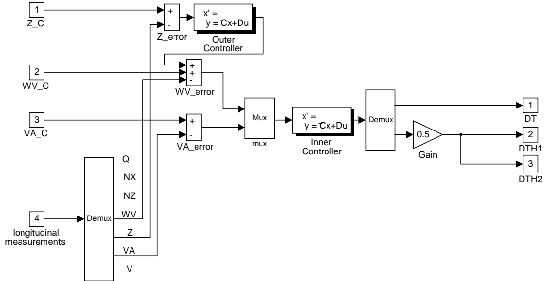
Figura 7: Estructura del controlador longitudinal
